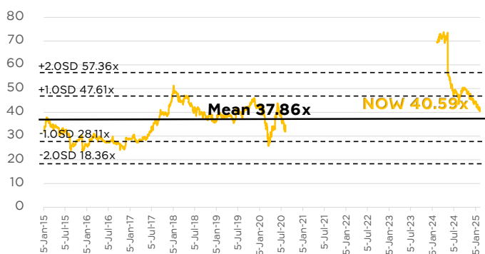
Fig. 4: AOT's Trailing PE
