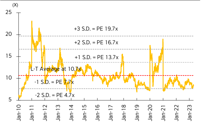
Figure 8: SAT PE
