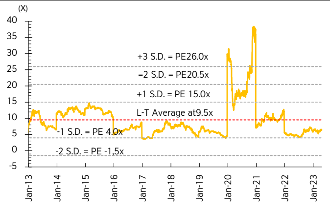
Figure 7: AH PE
