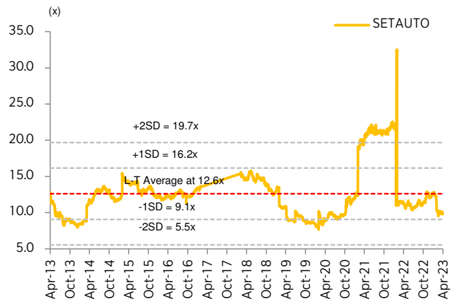
Figure 6: Auto PE
